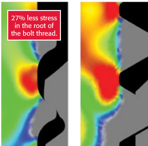
Huck 360®
